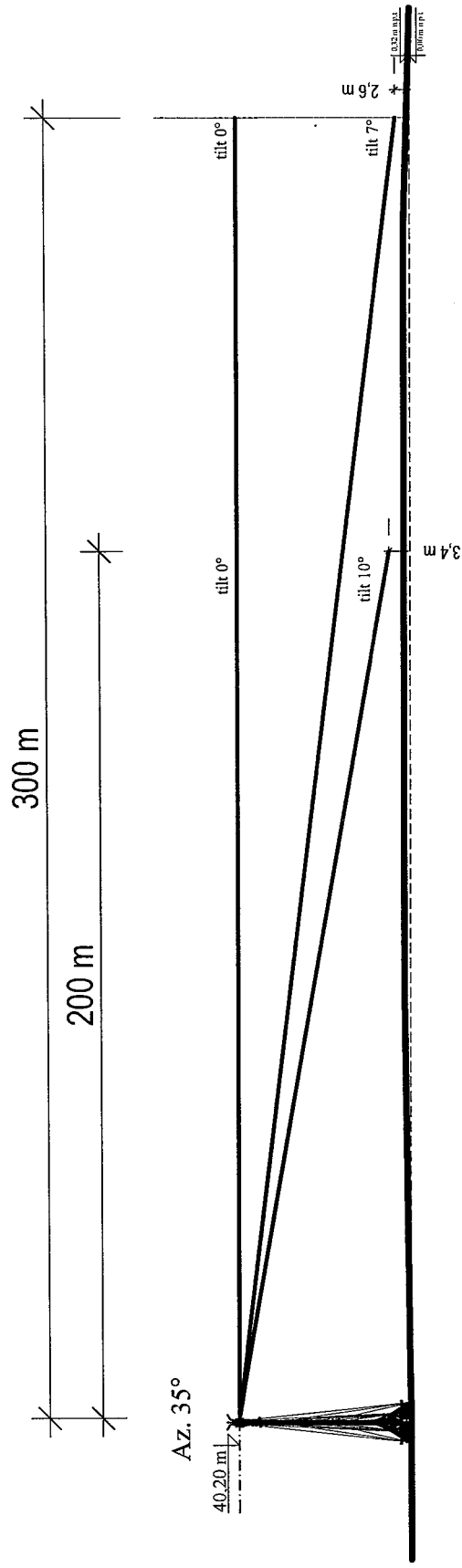
Rys. 2. Rzut pionowy osi głównej wiązki promieniowania na azymucie 35^\circ w odległości do 200 i 300 metrów od środka elektrycznego anteny sektorowej dla tiltów 0^\circ , 7^\circ oraz 10^\circ .
