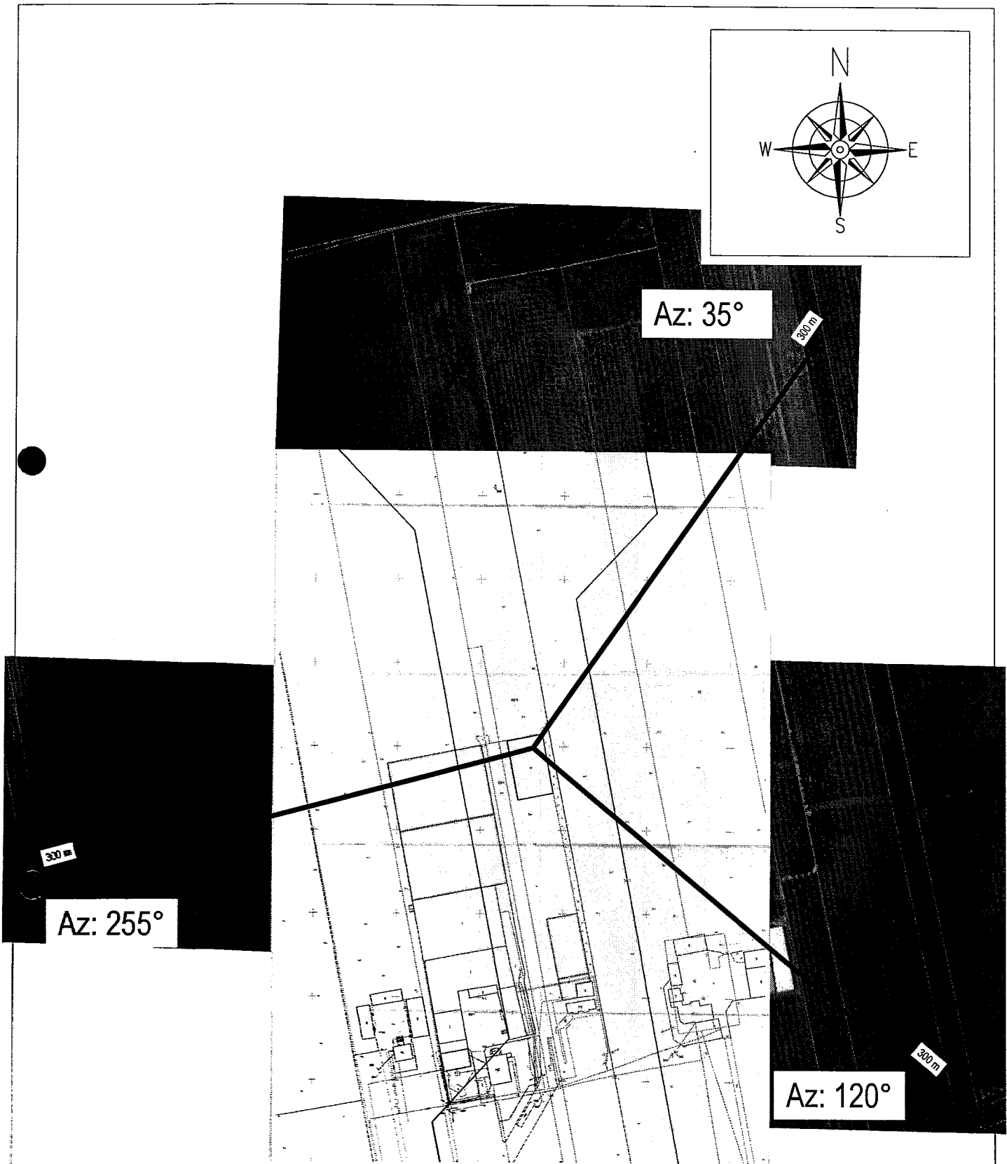
Rys. 1. Rzut poziomy osi głównej wiązki promieniowania w odległości do 200 i 300 metrów od środka elektrycznego anten sektorowych.
